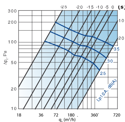
LK-200 (id=200mm)
