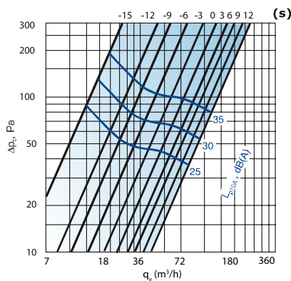
LK-080 (id=80 mm)
