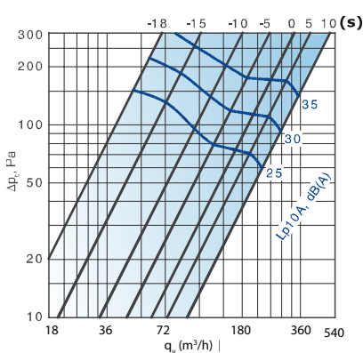
LK-160 (id=160mm)
