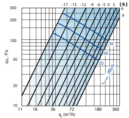
LK-125 (id=125 mm)
