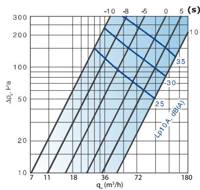
LK-100 (id=100 mm)
