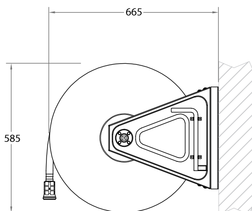
Vy sidan
