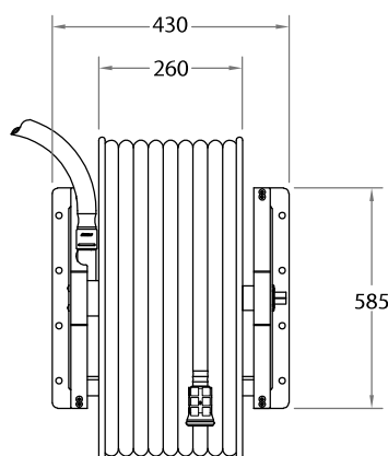
Vy framifrån
